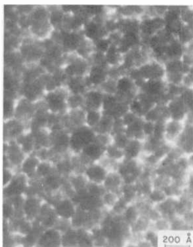
B. TEM OF SPUTTERED INCONEL 600
